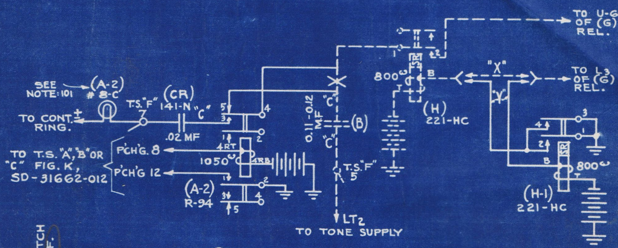
FIG. 2 WIRING DIAGRAM
